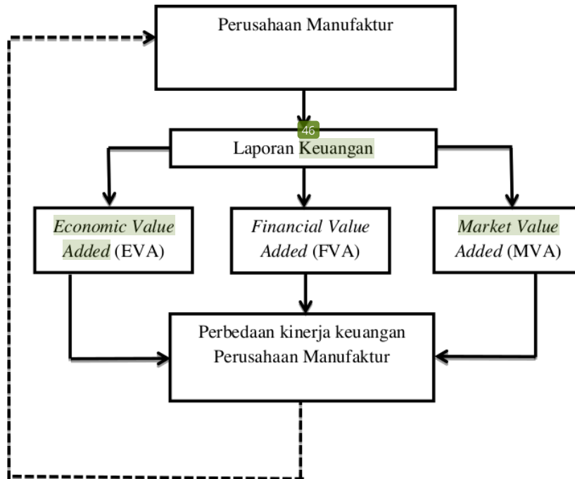
Gambar 2.1. Kerangka Konseptual
