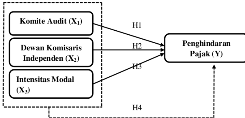
Gambar 2.1. Kerangka Konseptual
