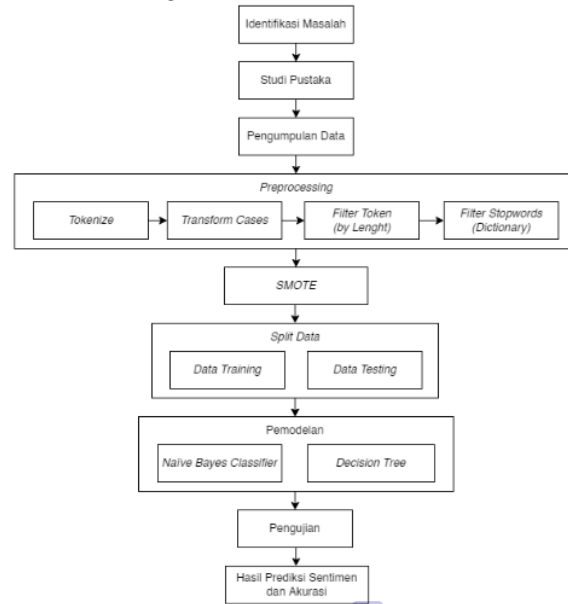
Gambar 1. Metodologi Penelitian
